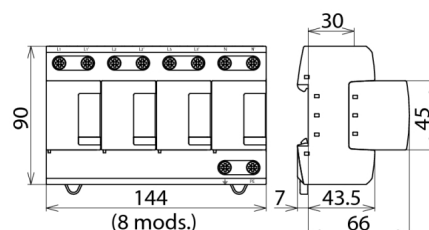
Rysunek wymiarów DV M TNS 255
