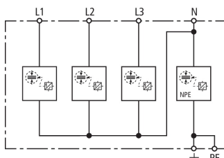
Schemat połączeń DSH TT 255
