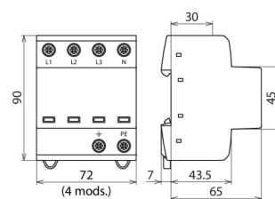
Rysunek wymiarowy DSH TT 255
